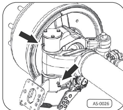
Rys. 13 • Punkty smarowe sworznia zwrotnicy
