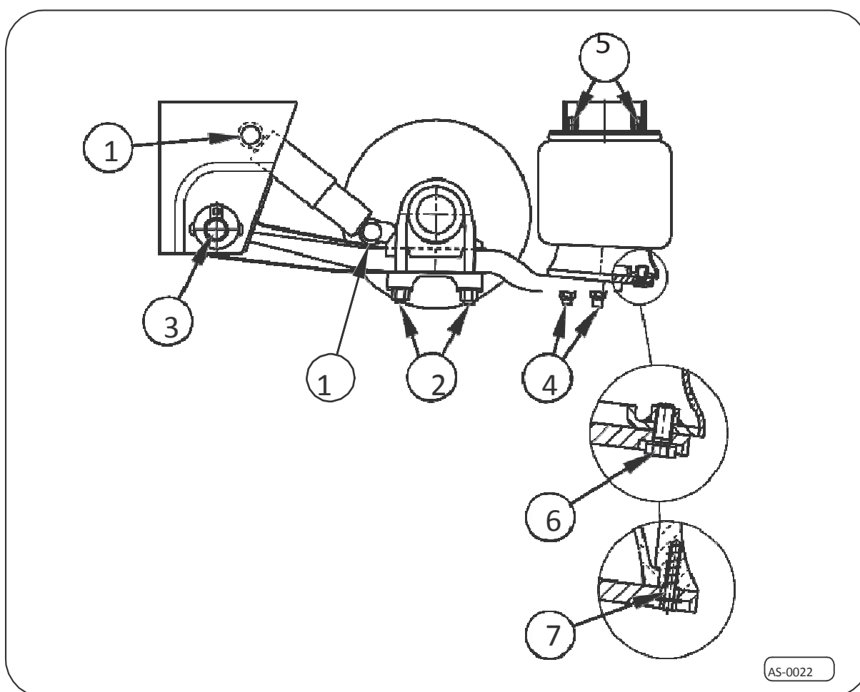
Rys. 9 • Wymagane kontrolne momenty dokręcenia SAF MODUL
